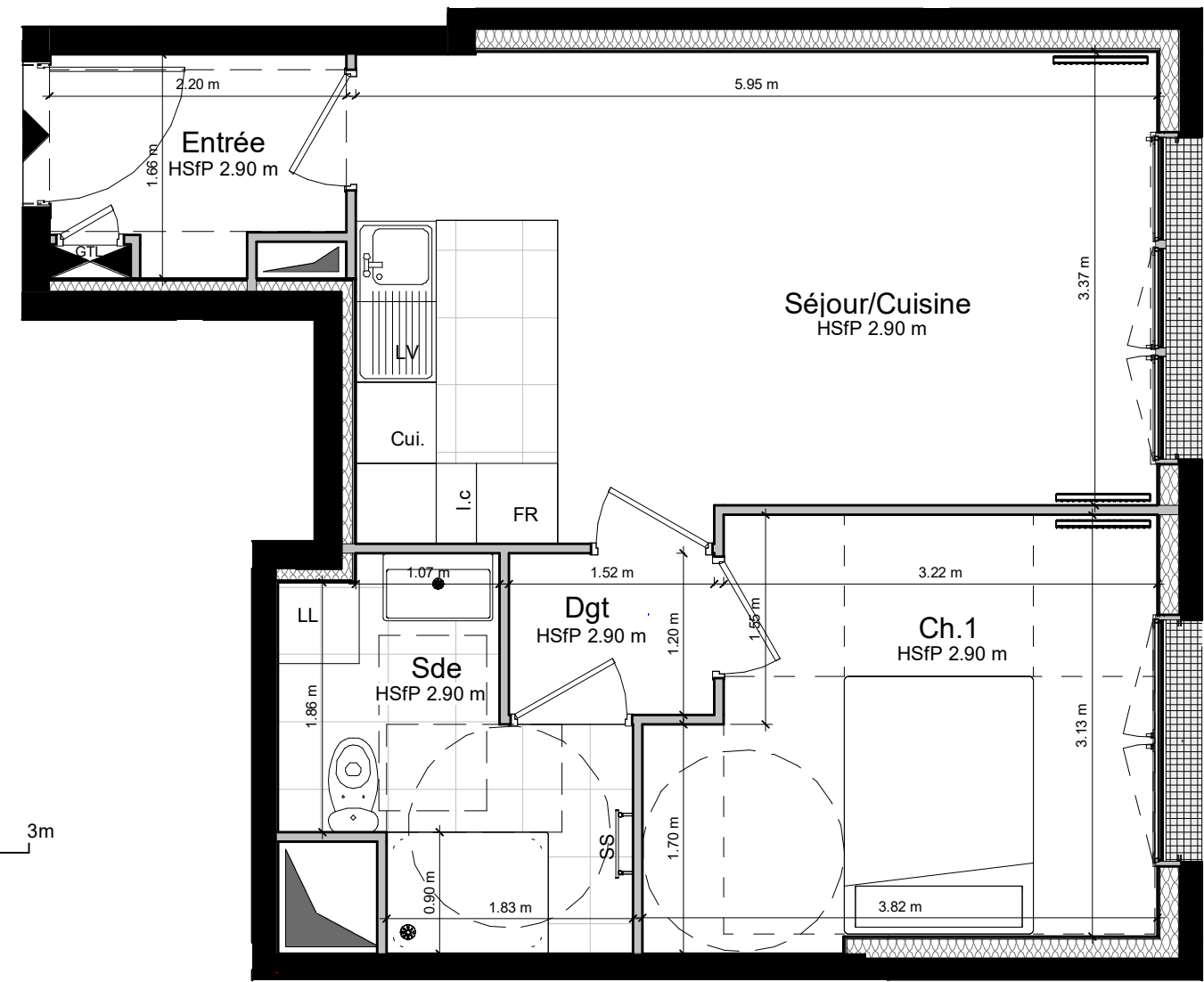
2 02-RDC - PDV - 001 Agrandi 1 : 50
