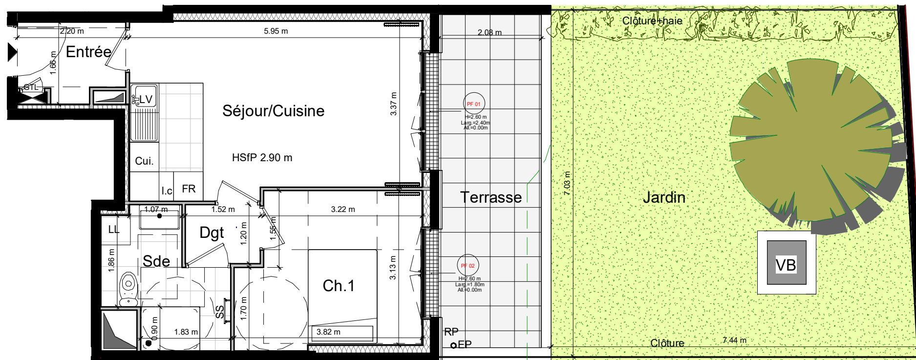
1 02-RDC - PDV - 001 1 : 75
